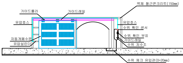
- 수문개폐 구조도 -
