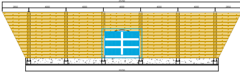
- 반수면부 정면도 -
