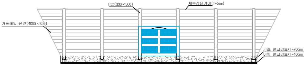
- 대수면부 정면도 -
