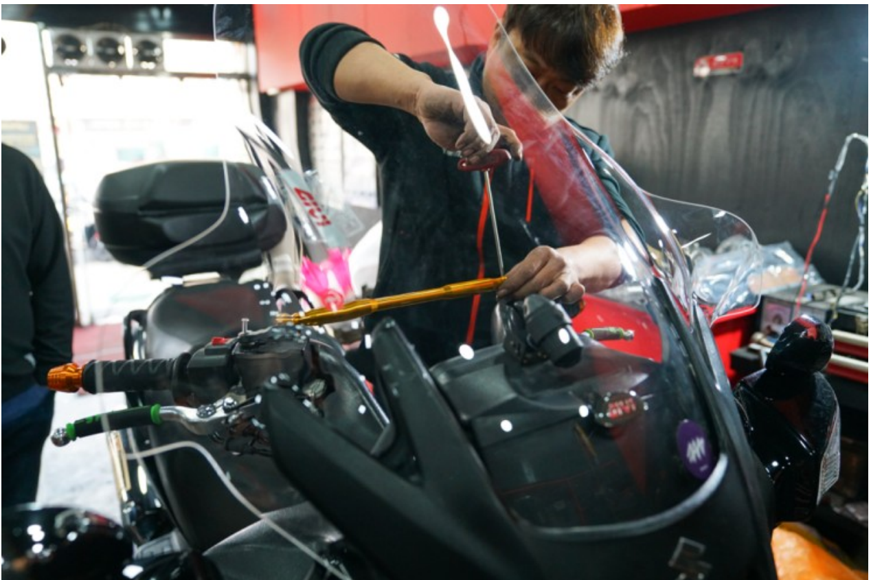
버그만650 구형은 좌우 마스터실린더캡의 높이가 약간 다르기 때문에 양 옆을 봐가며 핸들바를 조금씩 고정해 들어가야 합니다. 한쪽부터 모두 고정하고 시작하면 마스터 실린더 캡에서 브레이크액이 누유 될 수 있습니다.
