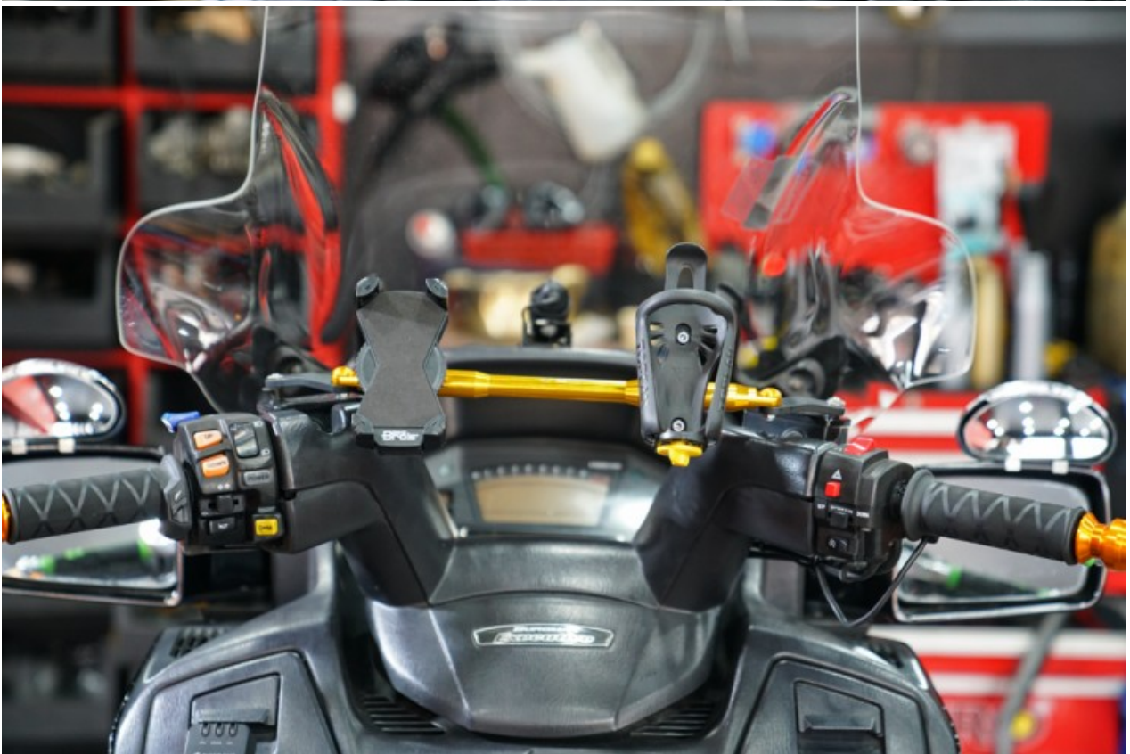
버그만650에 장착이 완료된 핸들바의 모습입니다. 좌우 균형이 맞도록 정확하게 최대한 중심을 잡아 견착하였습니다.
